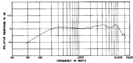
60Hz A 15000 KHz gráfico de resposta de freqüência
