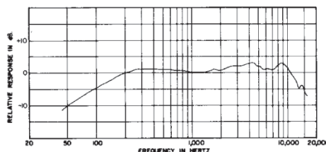
60Hz A 15000 KHz gráfico de resposta de frequência
